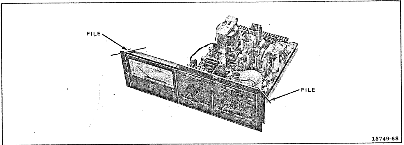
Figure 7-1. I/O Module
